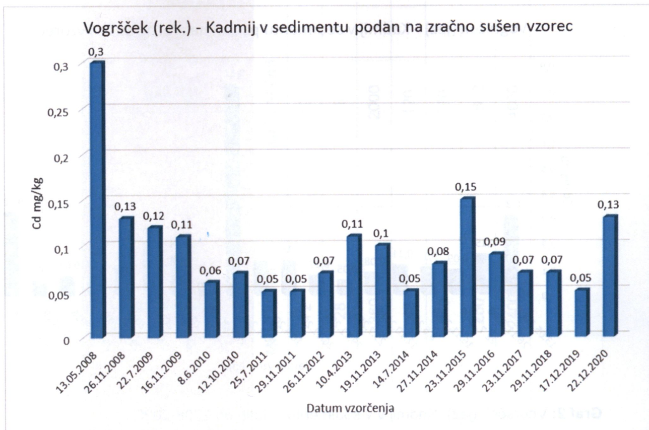
Graf 4: Vogršček (rekreacijski del): Kadmij v sedimentu, v letih od 2008-2020
