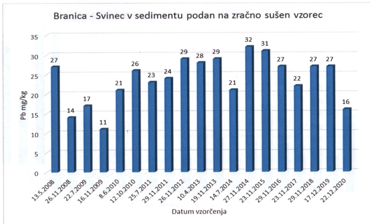
Graf 8: Branica: Svinec v sedimentu, v letih od 2008-2020
