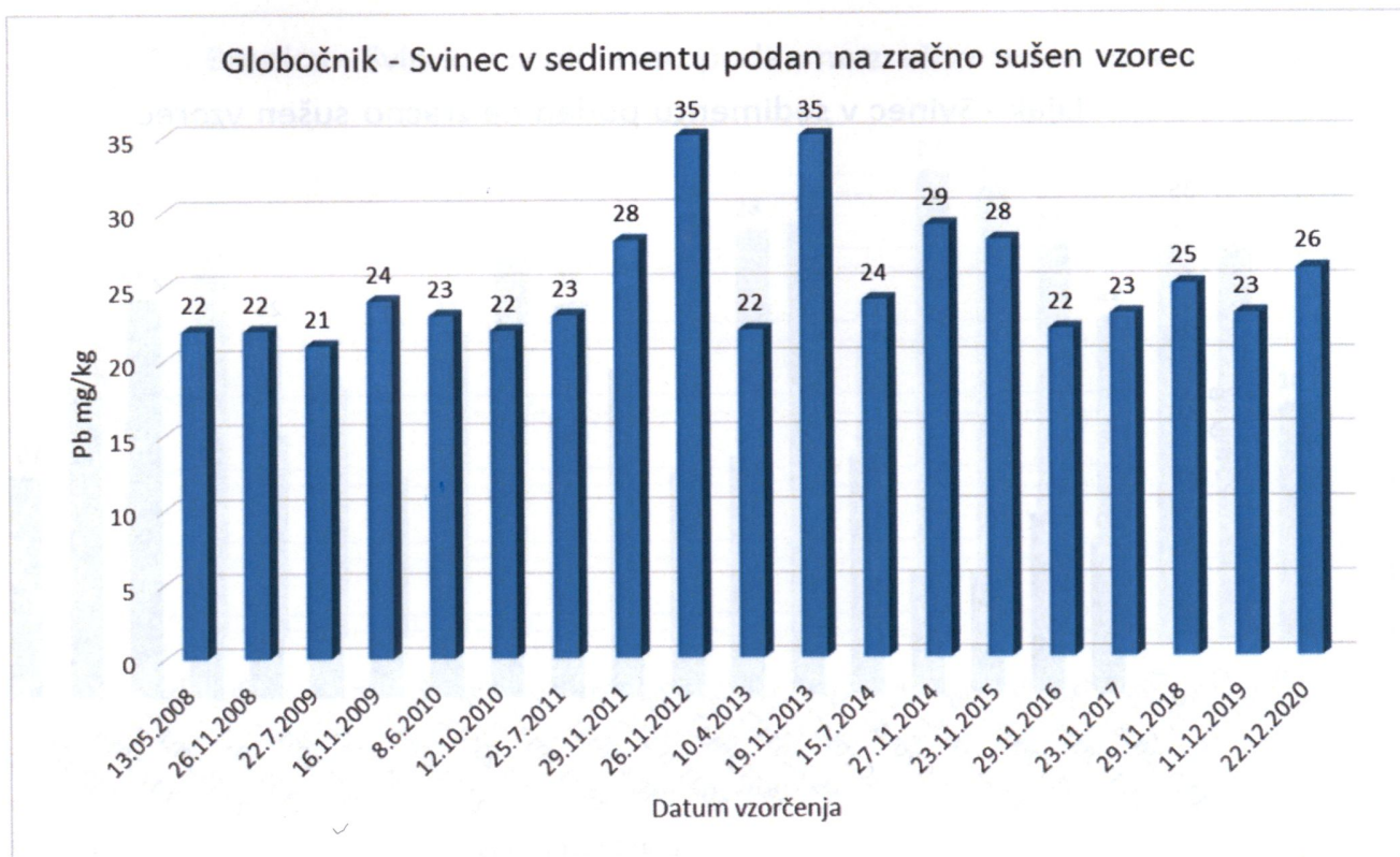
Graf 12: Globočnik: Svinec v sedimentu, v letih od 2008-2020
