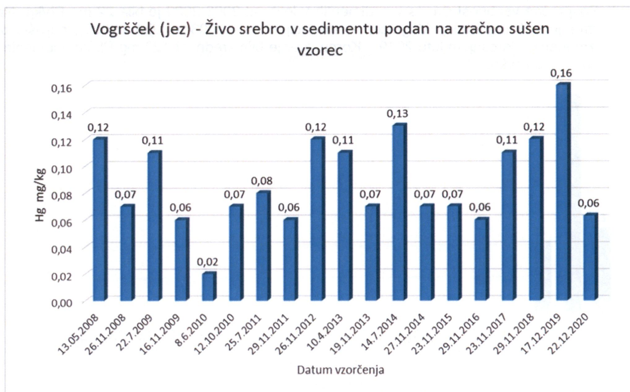
Graf 16: Vogršček (jez): Živo srebro v sedimentu, trend v letih od 2008-2020
