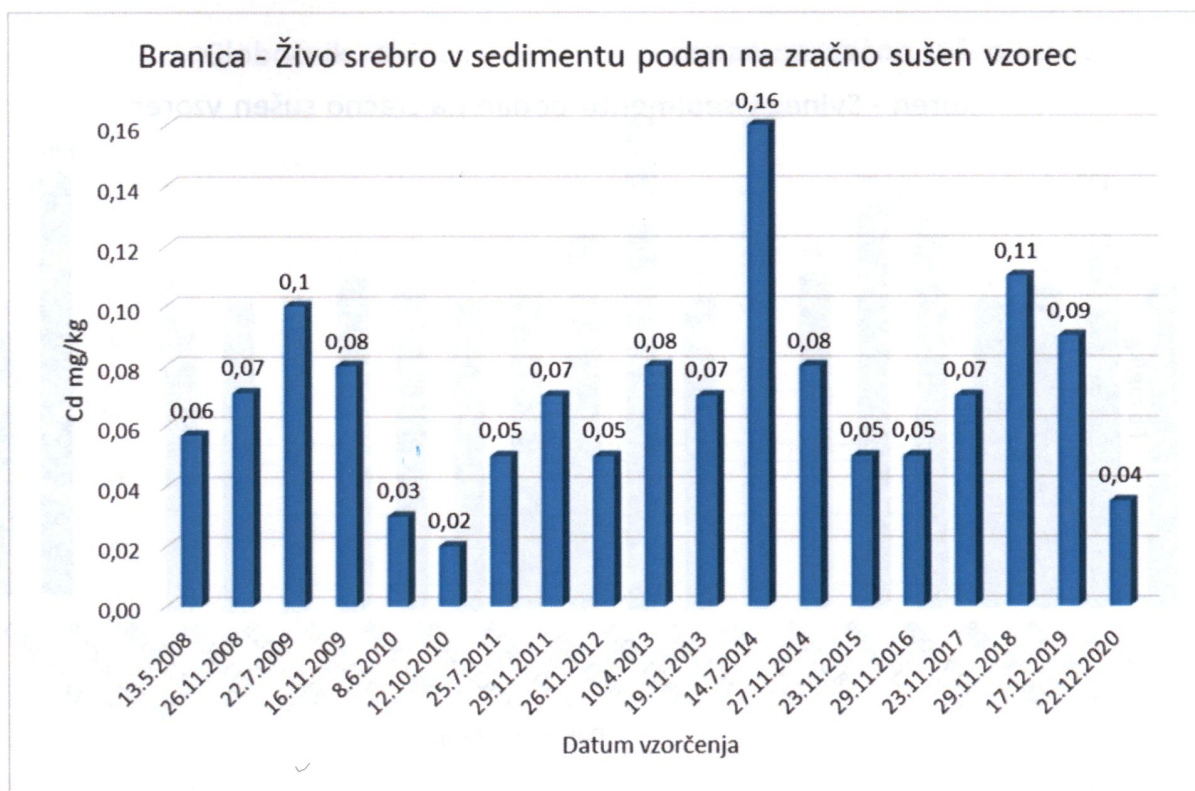
Graf 15: Branica: Živo srebro v sedimentu, trend v letih od 2008-2020
