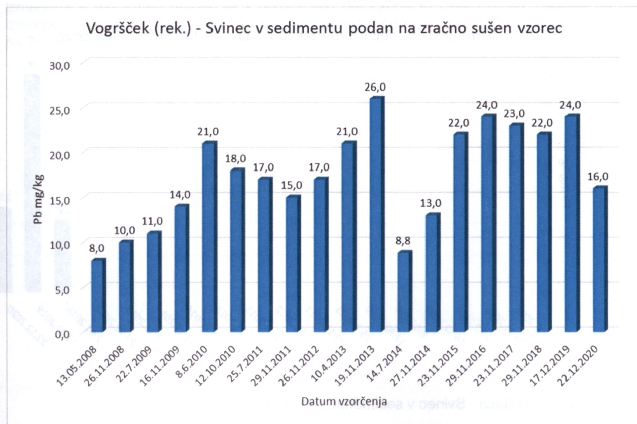
Graf 11: Vogršček (rekreacijski del): Svinec v sedimentu, v letih od 2008-2020
