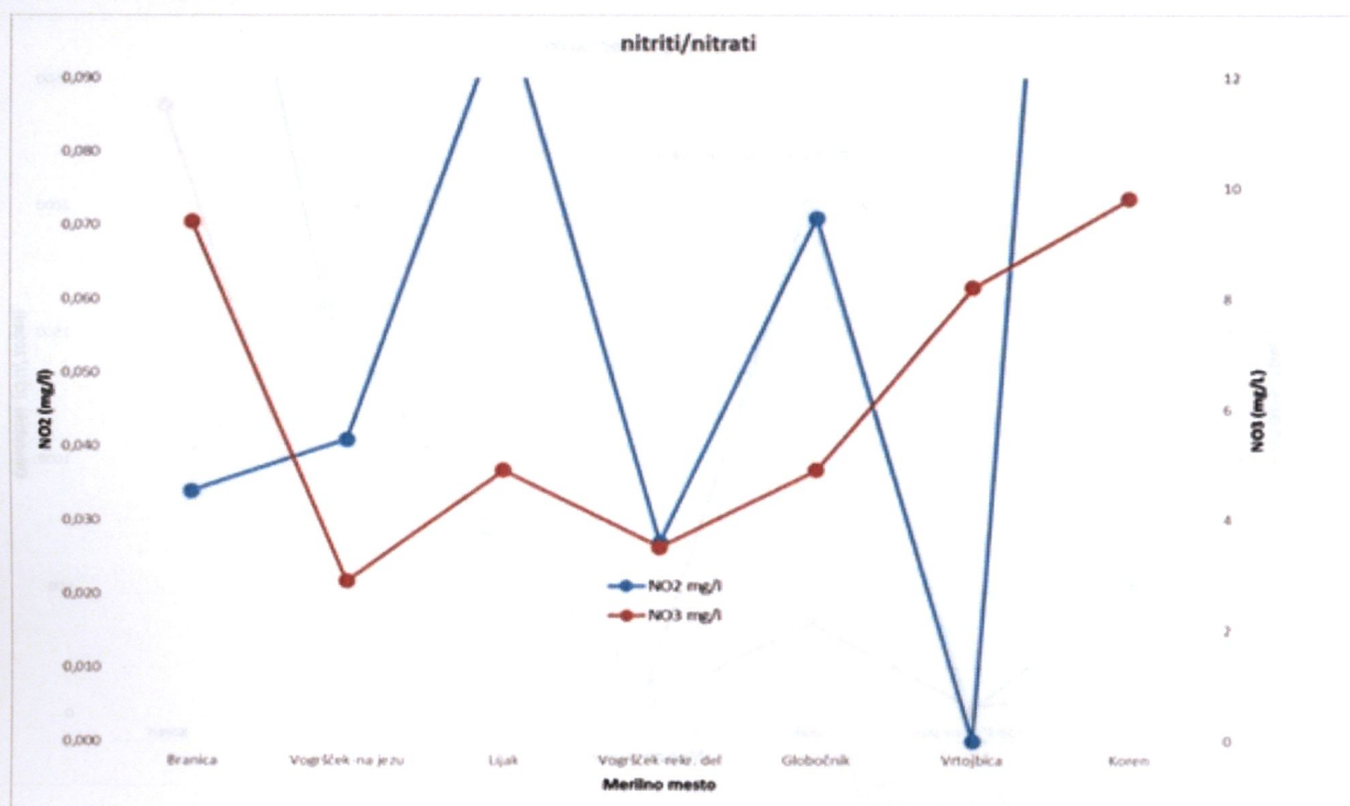
Graf 23: Vsebnost nitritov in nitratov
