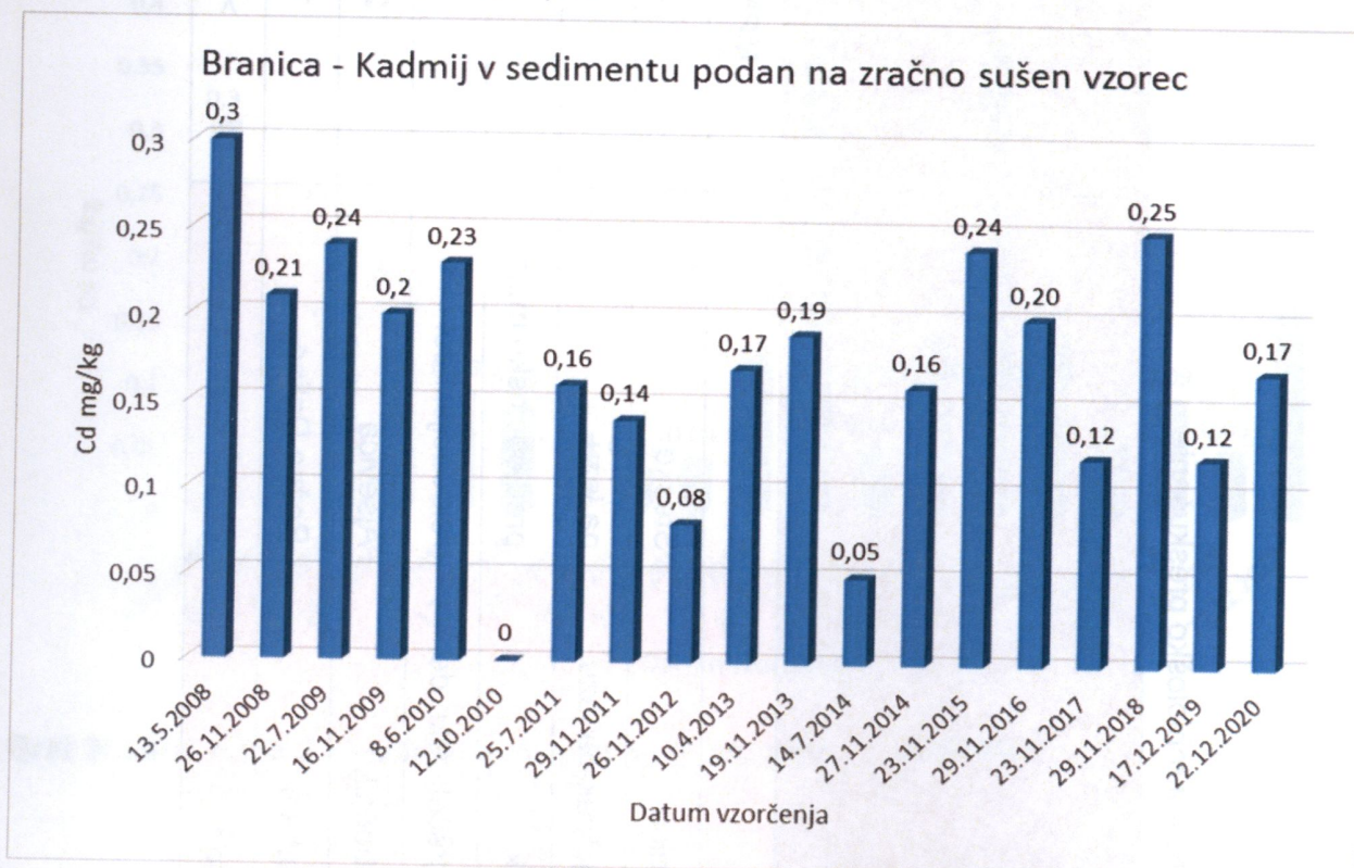
Graf 1: Branica: Kadmij v v sedimentu, v letih od 2008-2020
