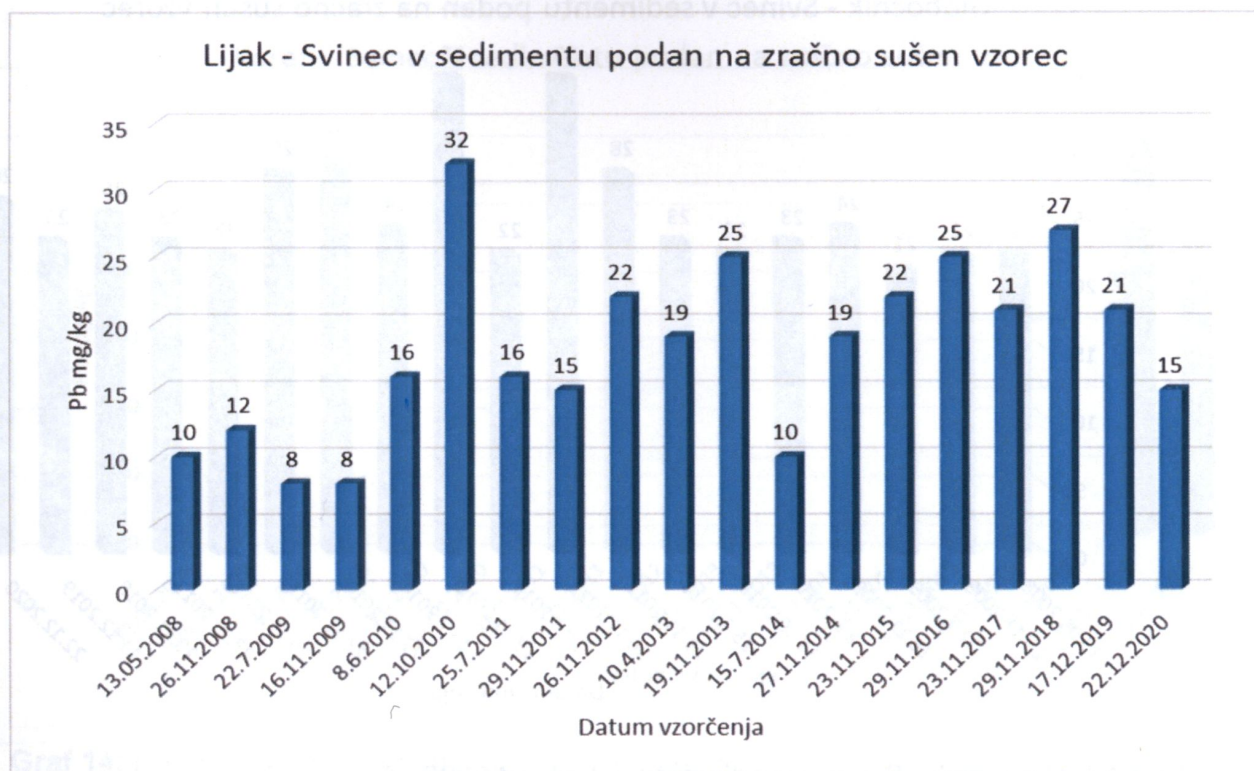
Graf 10: Lijak: Svinec v sedimentu, v letih od 2008-2020
