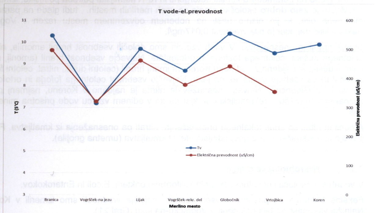
Graf 22: Temperature vode in električna prevodnost
