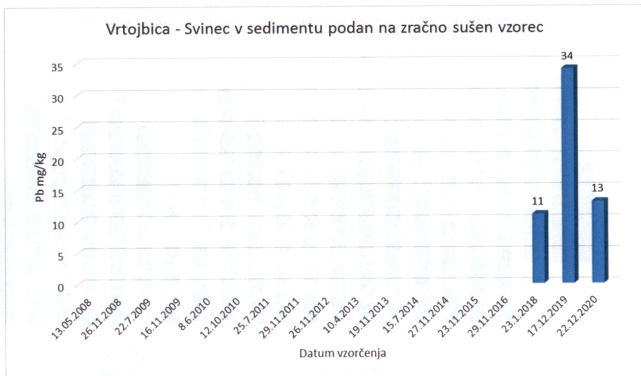
Graf 13: Vrtojba: Svinec v sedimentu, v letih od 2008-2020
