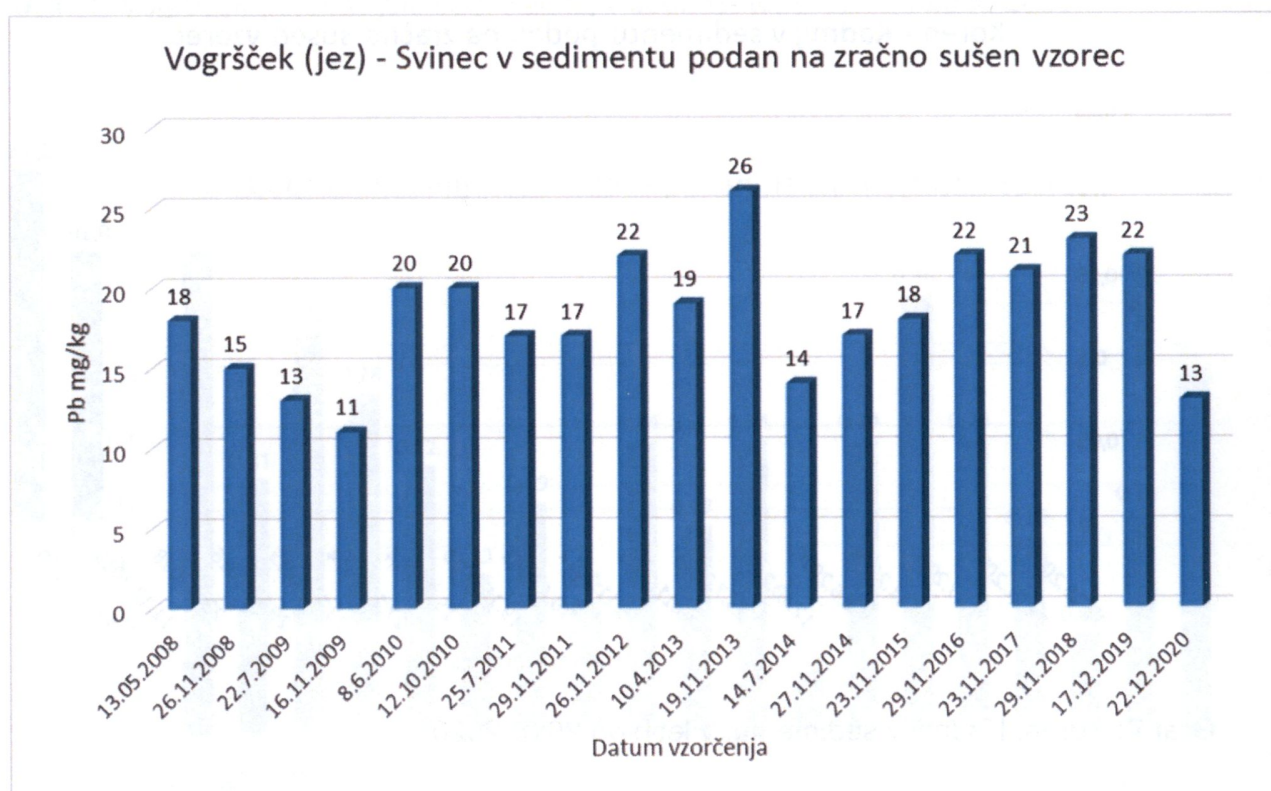
Graf 9: Vogršček (jez): Svinec v sedimentu, v letih od 2008-2020
