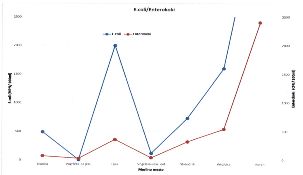
Graf 21: Mikrobiološke preiskave
