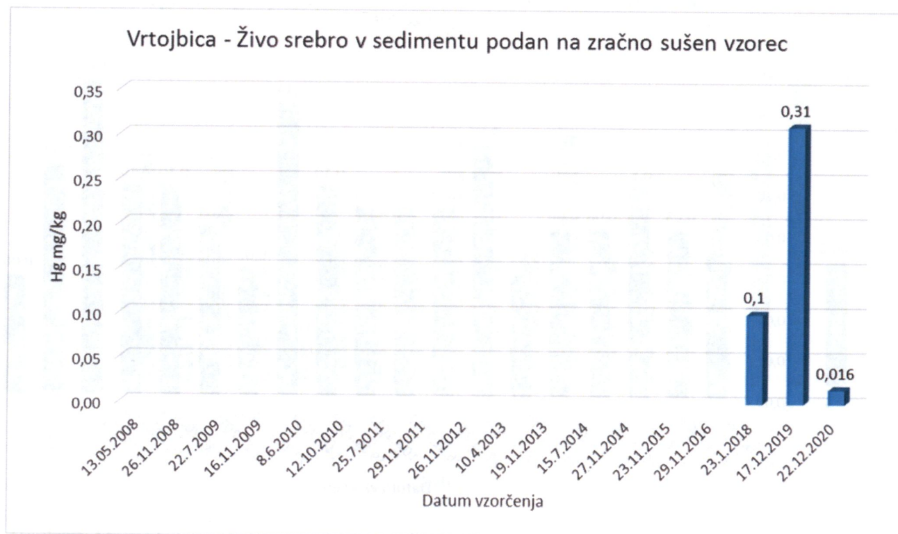
Graf 20: Vrtojba: Živo srebro v sedimentu, trend v letih od 2018-2020
